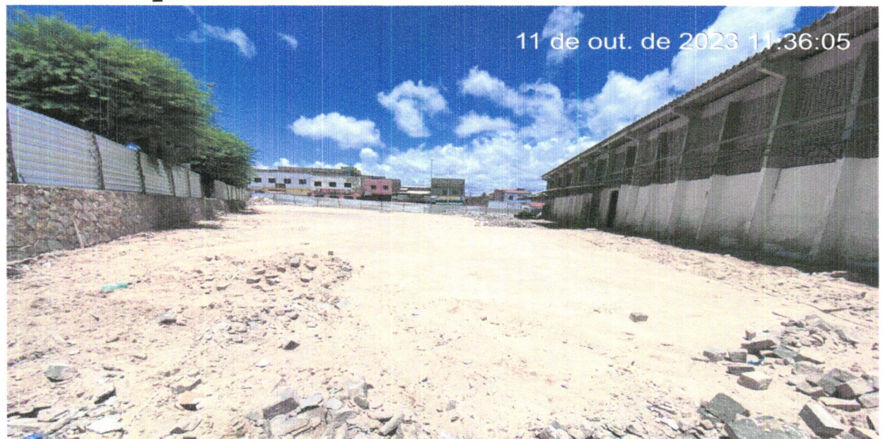
FOTO 30 - ATERRO MANUAL DE VALAS COM SOLO ARGILO-ARENOSO E COMPACTAÇÃO MECANIZADA. AF_05/2016
